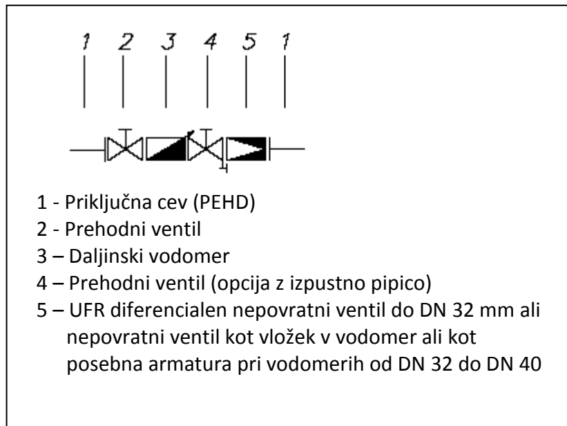
PRILOGA št. 4: Slika 1: Merilno mesto priključka do DN 40 (sestav in zaporedje obveznih elementov)
