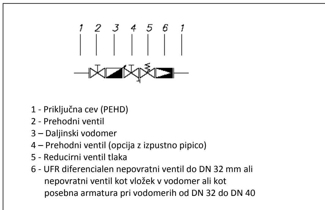
PRILOGA št. 4: Slika 2: Merilno mesto priključka do DN 40 z reducirnim ventilom tlaka (sestav in zaporedje obveznih elementov)
